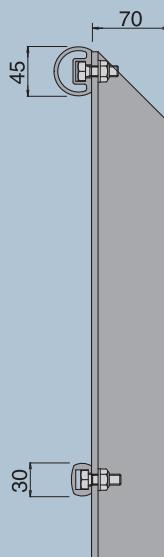
a部詳細図
