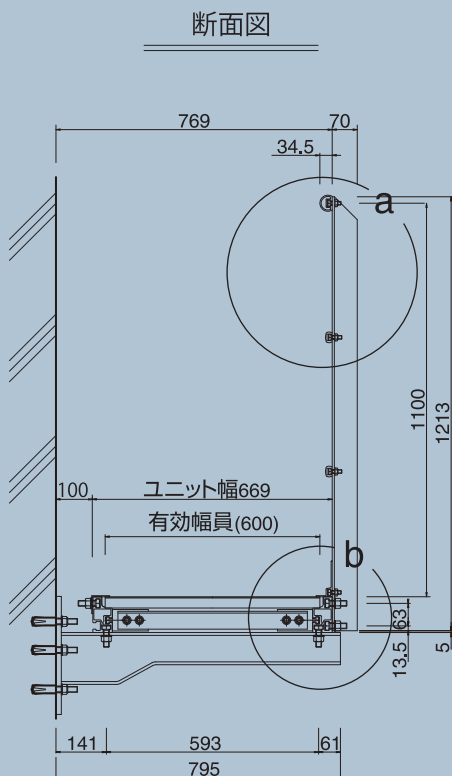
床版パネル断面図
