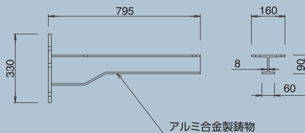
下部工ブラケット標準図
