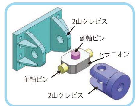
U-CLV の構造
