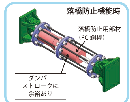
落橋防止用部材を増設した構造
