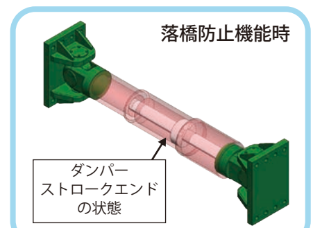
ダンパー本体が直接抵抗する構造
